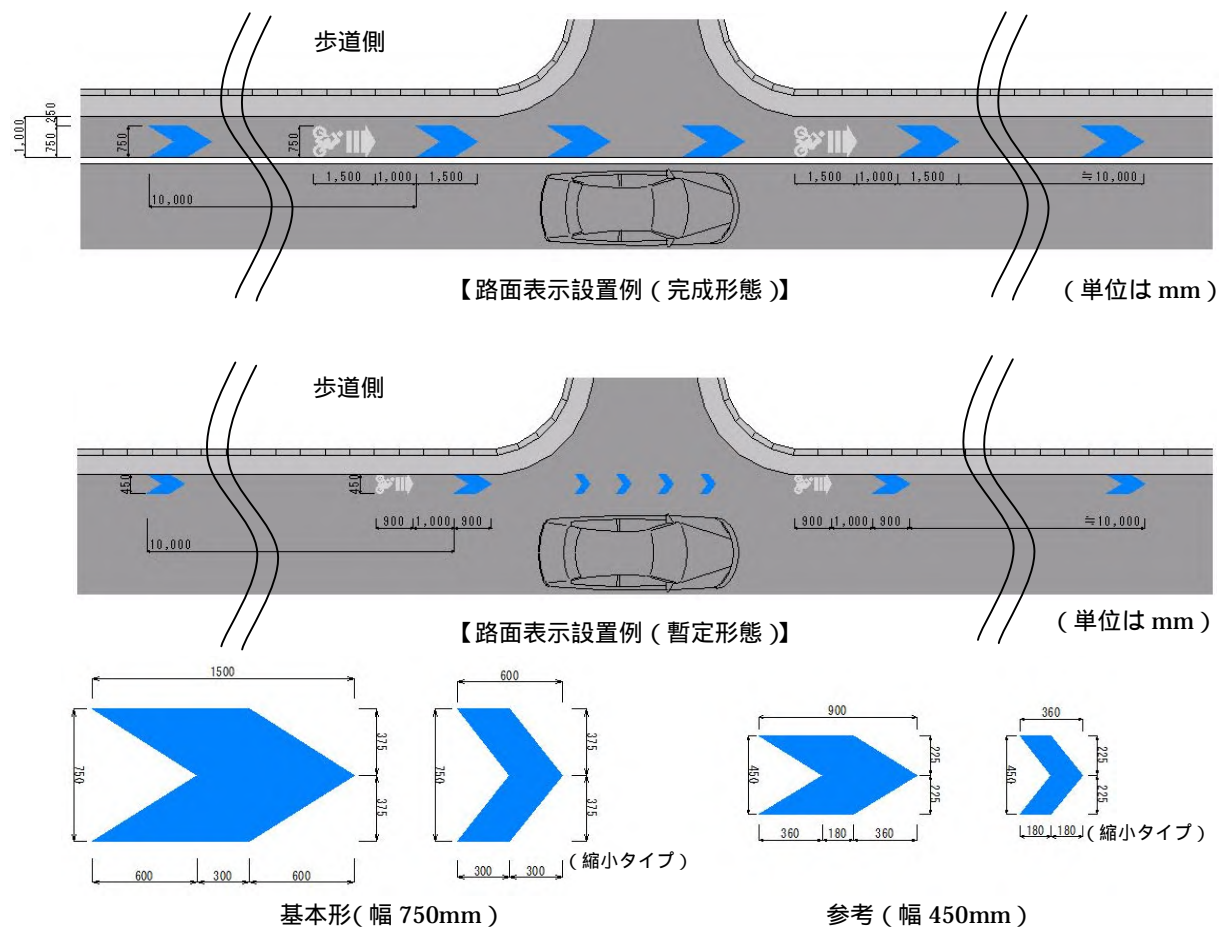
図 5-6 車道混在パターンの法定外路面表示
