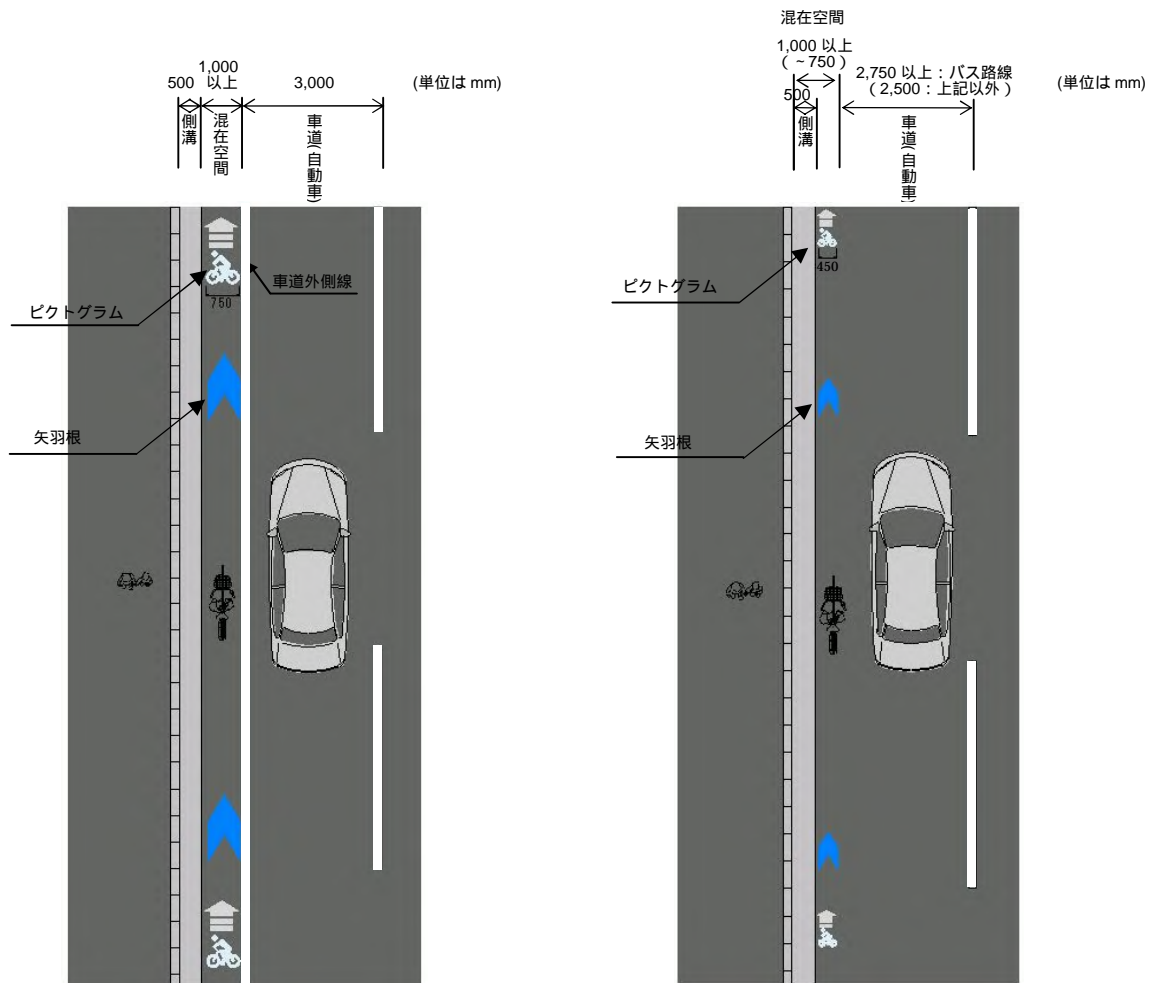
図 4-11 完成形態（車道混在）
