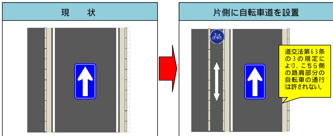
図 4-4 片側に歩道が設置された一方通行の場合の自転車道の設置 (条件を満たす特別の場合に限り、暫定的に双方向通行を適用)
