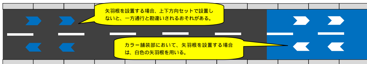
図 5-1 自転車道への矢羽根の設置例
