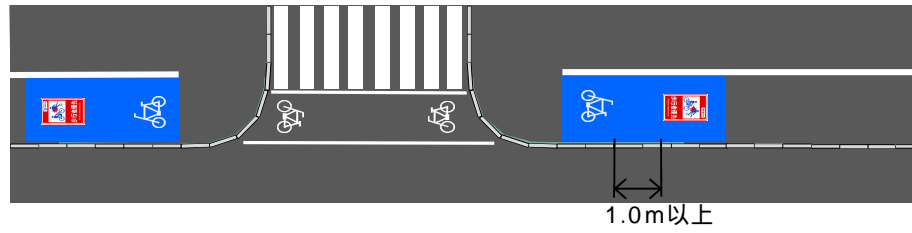
図 5-24 啓発サインと注意喚起サインの離隔
