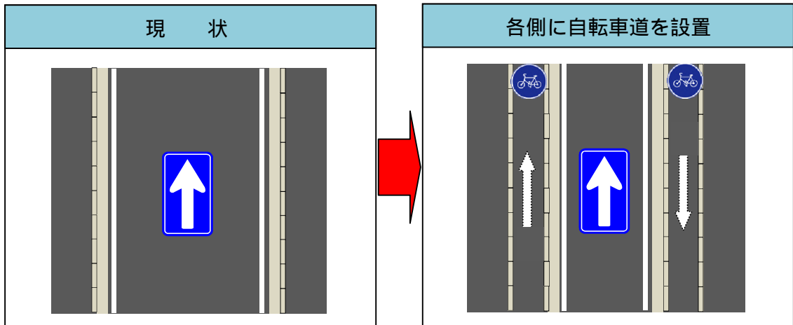
図 4-3 各側に歩道が設置された一方通行の場合の自転車道の設置 (自転車道は一方通行を基本)
