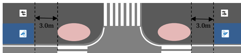
図 5-11 自転車の走行位置の法定外の明示を行わない場所（交差側の横断方向の手前）
