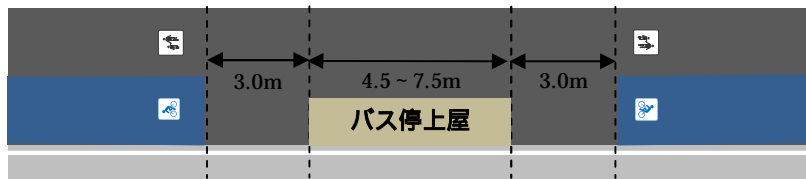
図 5-12 自転車の走行位置の法定外の明示を行わない場所（バス停の手前）
